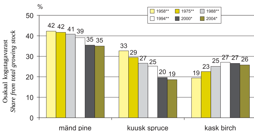
Joonis 1.6.1.2 Puuliikide osakaalu muutumine
