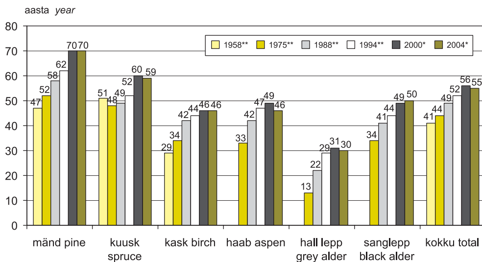
Joonis 1.8.1.1 Puistute keskmise vanuse muutumine
