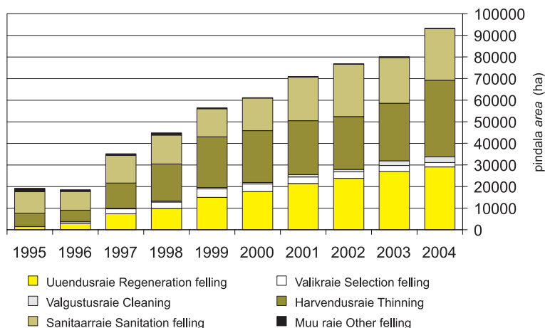
Joonis 3.3.6.1 Raiete pindala raieliigiti erametsamaal aastail 1995–2004
