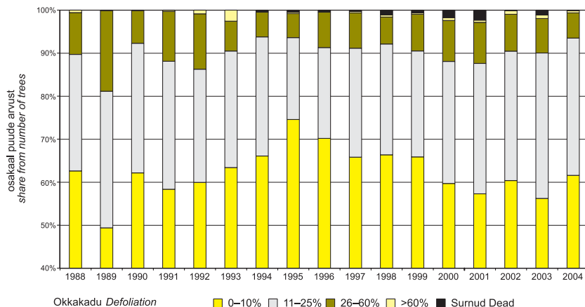
Joonis 5.7.1 Hariliku kuuse okkakadu metsaseire proovipunktides aastail 1988–2004 Figure 5.7.1 Defoliation of Norway spruce on forest monitoring sample points in 1988–2004
