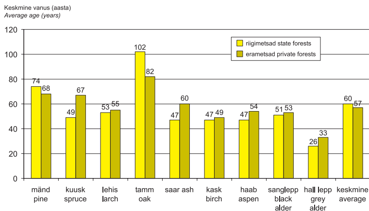
Joonis 1.8.2.1 Puistute keskmine vanus
