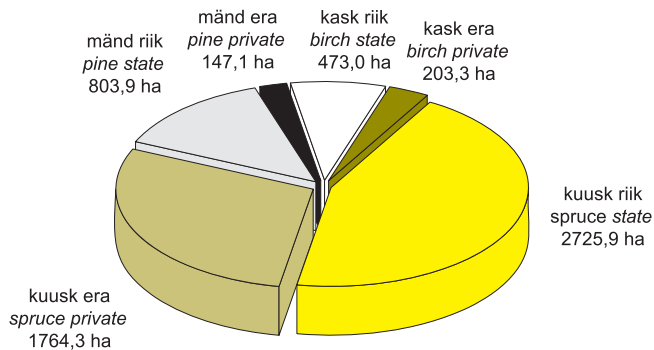
Joonis 4.2.4.1 Metsaistutus riigi- ja erametsas puuliikide lõikes pinna järgi 2004. aastal
