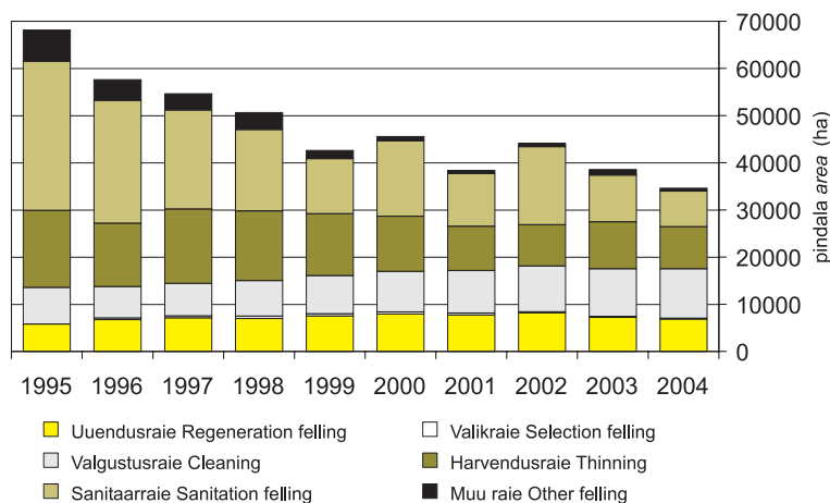
Joonis 3.3.4.1 Raiete pindala raieliigiti riigimetsamaal aastail 1995–2004
