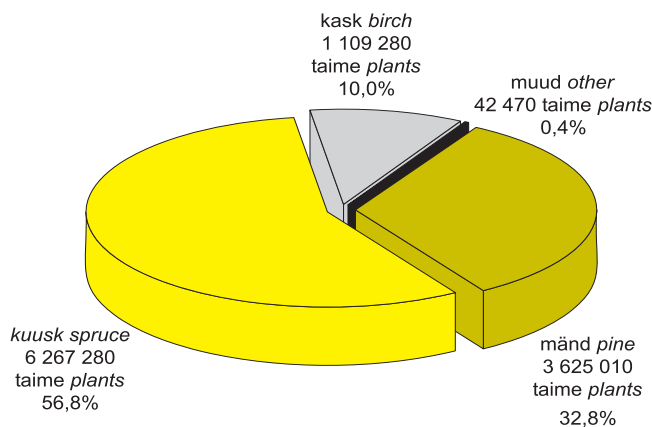
Joonis 4.2.4.3 Metsaistutus riigimetsas puuliikide lõikes taimede arvu järgi 2004. aastal
