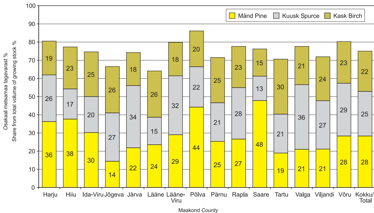
Joonis 1.6.2.3 Männipuidu, kuusepuidu ja kasepuidu osakaal metsamaa tagavarast maakonniti
