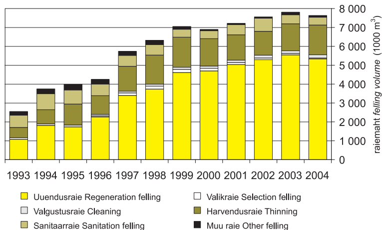
Joonis 3.3.2.1 Raiemaht raieliigiti aastail 1993–2004
