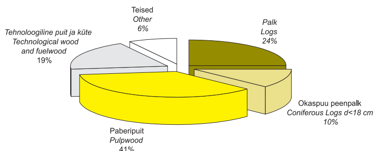
Joonis 10.4.2.1.1 2004. aastal ümarmaterjalidena müüdud puidukoguse jagunemine sortimentideks
