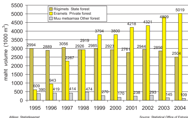
Joonis 3.4.1 Raiemahu jagunemine metsamaaomanike järgi aastail 1995–2004
