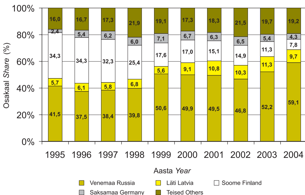
Joonis 10.3.3.2 Suurimate väliskaubanduspartnerite osakaal puidu ja puittoodete (kaubajaotus 44) koguimpordist aastail 1995–2004
