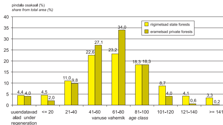
Joonis 1.11.2.1 Männikute metsamaa pindala jagunemine vanuse järgi
