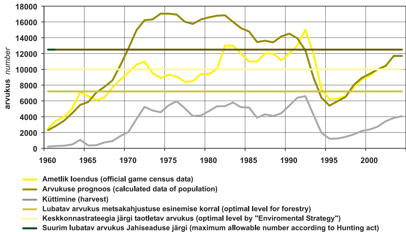
Joonis 8.4.1.1 Põdra arvukus ja küttimine aastail 1960–2004
