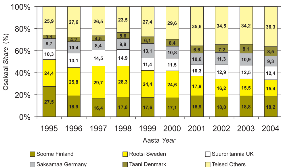
Joonis 10.3.3.1 Suurimate väliskaubanduspartnerite osakaal puidu ja puittoodete (kaubajaotus 44) kogueksportist aastail 1995–2004
