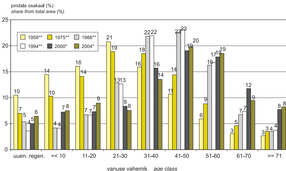
Joonis 1.13.1.1 Kaasikute vanuselise jagunemise muutumine
