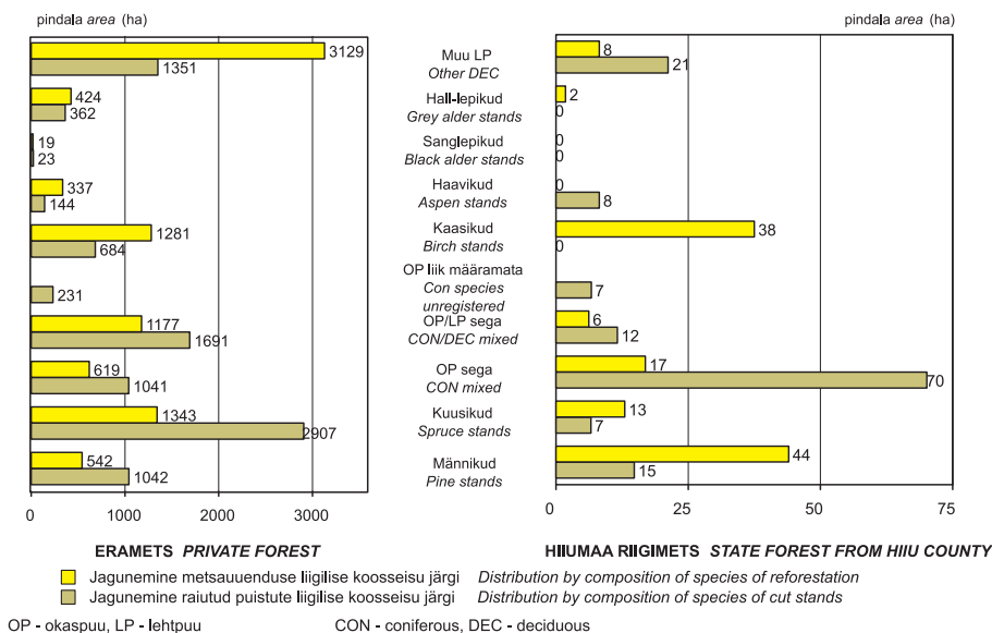
Joonis 4.5.2 Uuenemiseks eeldusi omavate lageraie alade jagunemine liigilise koosseisu järgi puistutes enne raiet ja 4. aastal pärast raiet
