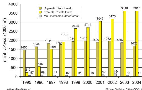
Joonis 3.4.2 Uuendusraie mahu jagunemine metsamaaomanike järgi aastail 1995–2004
