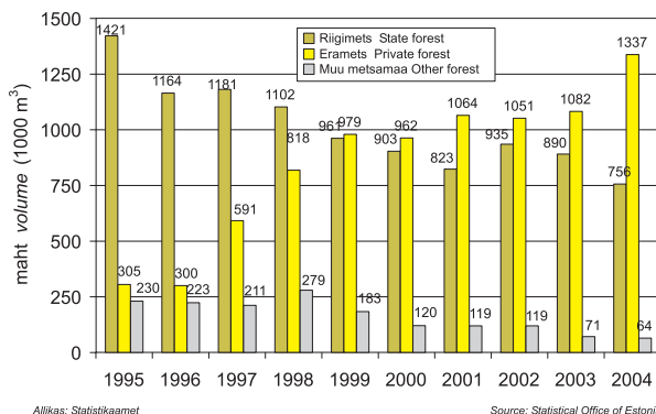
Joonis 3.4.3 Hooldusraiete mahu jagunemine metsamaaomanike järgi aastail 1995–2004
