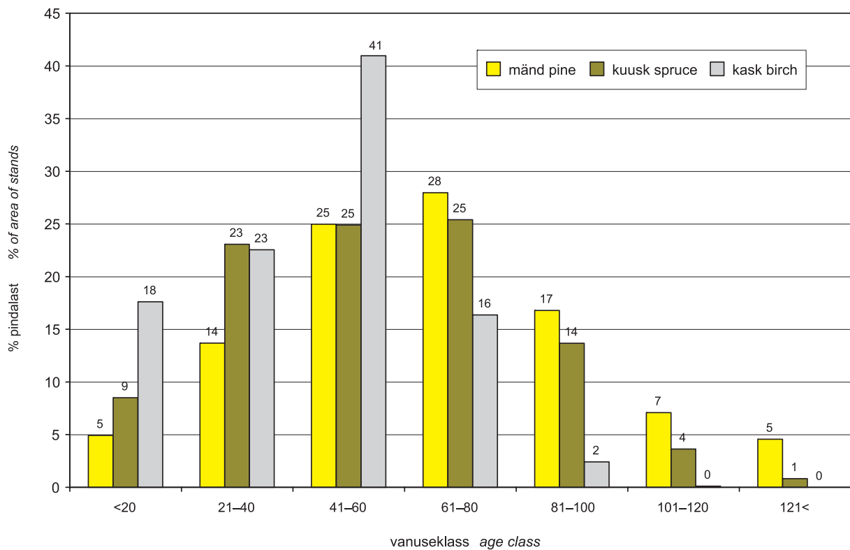
Joonis 1.3.2.1 Puistute jagunemine vanuseklassidesse enamuspuuliigi järgi Figure 1.3.2.1 Distribution of stands by age classes and dominant tree species
