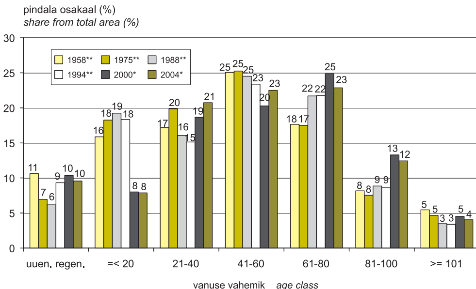
Joonis 1.12.1.1 Kuusikute vanuselise jagunemise muutumine
