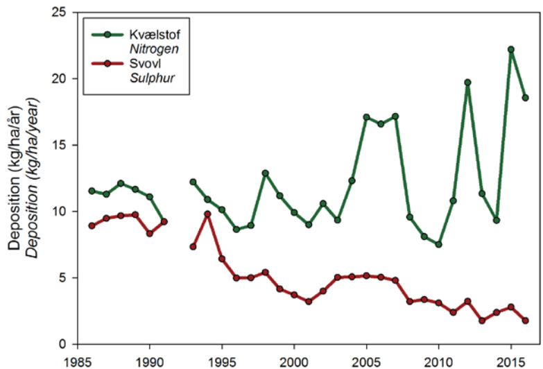
Figur 2.1. Udviklingen i tilførslen (depositionen) af svovl (sulfat) og kvælstof (nitrat og ammonium) fra 1986 til 2016 i bøgebevoksning ved Stenholt Vang i Nordsjælland. Tallene for svovl er korrigeret for det naturlige nedfald af sulfat-svovl fra havsalt, der blæser ind over land. En ændring i procedurerne for indsamling af prøver i 2002 kan have haft indflydelse på resultaterne.
